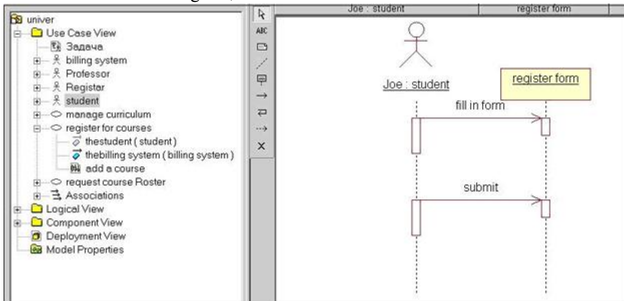
Рис. 6. Диаграмма последовательностей
