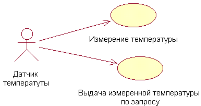
Рис.1. Диаграмма прецедентов
