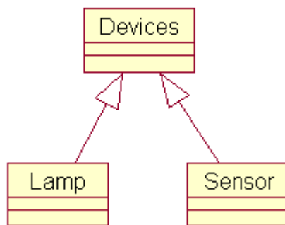
Рис.7. Диаграмма классов
